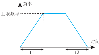
6-04 直线加减速
