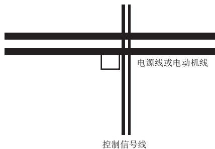
图3-26 系统配线要求
