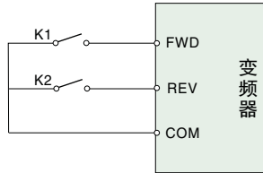
图6-20 两线式运转模式2
