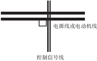
图3-17 系统配线要求
