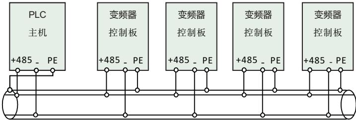
图3-14 PLC与变频器多机通信时的接线图（变频器、电机全部良好接地）
