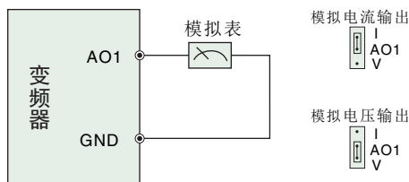
图3-11 模拟输出端子配线
