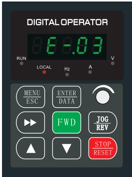
图4-5 故障警告显示状态
