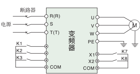
图6-16 多段速运行接线图
