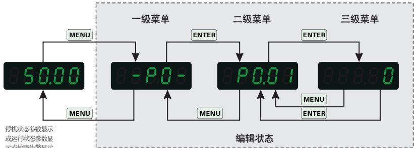
图4-6 操作面板编程显示状态
