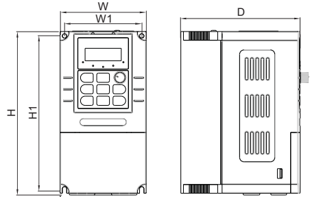
4T0007G-B~4T0075G-B外观尺寸图
