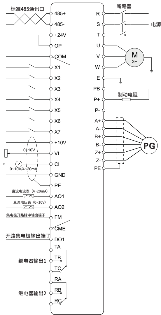
图3-7 基本配线图 （V9-4T0300G以上）
