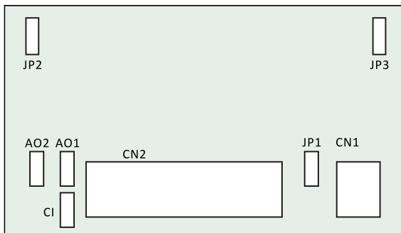
图3-7 控制板端子跳线位置示意图
