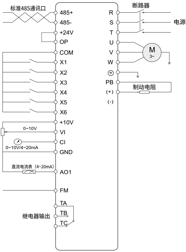
图3-5 基本配线图 (V9-4T0007G ~ V9-4T0075G)
