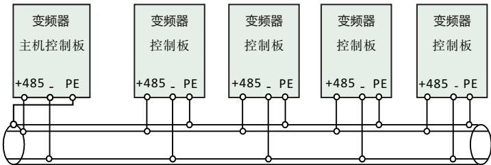
图3-15 变频器多机通信时的接线图（变频器、电机全部良好接地）
