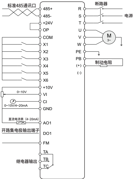
图3-4 基本配线图（V9-4T0007G-B ~ V9-4T0075G-B）
