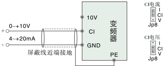
图3-10 CI端子配线图
