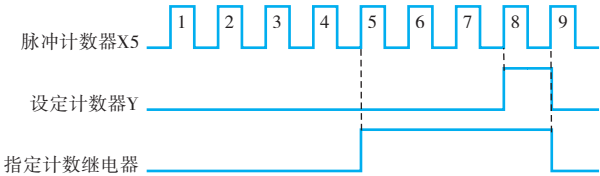
图6-37 设定计数值给定和指定计数值给定示意图
