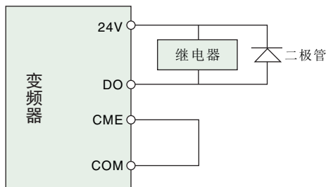
图3-12 数字输出端子配线示意图
