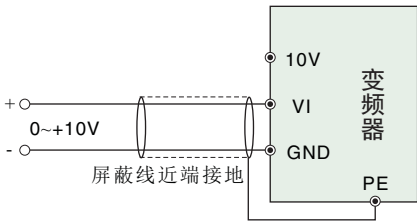
图3-9 VI端子配线图
