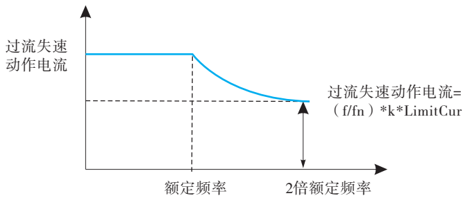
图6-38 倍速过流失速动作示意图
