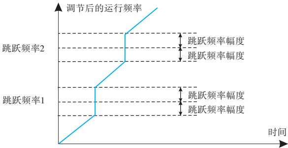
图6-10 加减速过程中跳跃频率有效示意图
