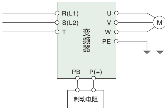
图2-9 变频器与制动组件连线图
