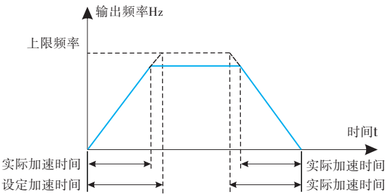
6-01 加减速时间示意图
