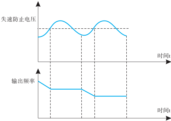
图6-33 过压失速功能
