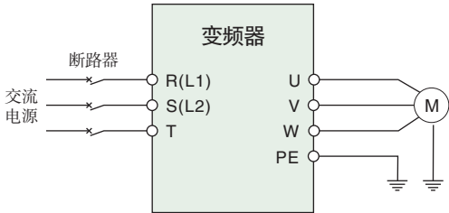
图3-3 主回路简单配线
