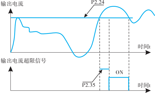
图6-14 输出电流超限检测示意图
