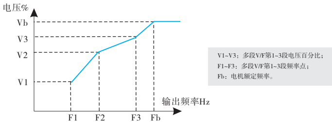
图6-25 多点V/F频率电压图
