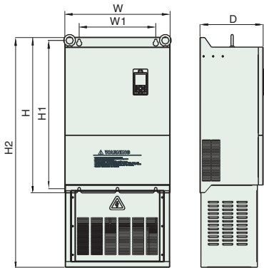
图2-6 加底座
