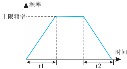
6-03 直线加减速
