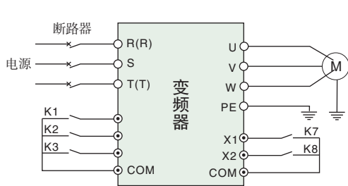
图6-16 多段速运行接线图
