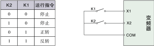
图6-20 两线式运转模式2
