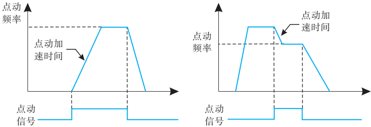
图6-05 点动运行
