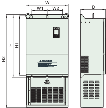
图2-8 加底座
