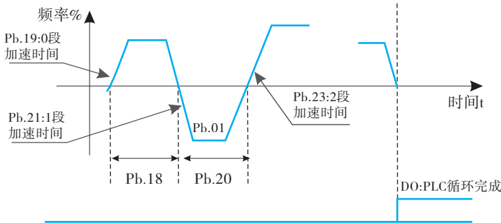
图6-35 简易PLC示意图
