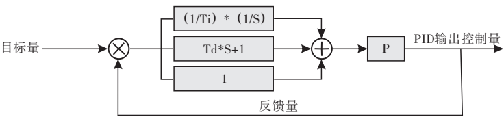
图6-26 过程PID原理框图
