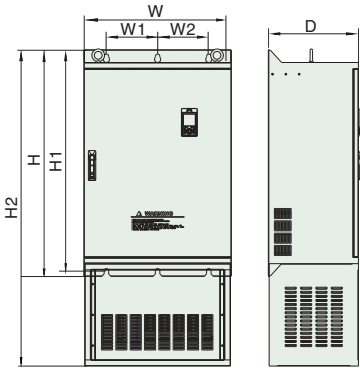
图2-10 加底座
