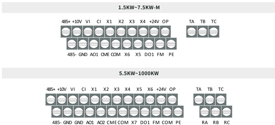
图3-6 控制板端子排列顺序图
