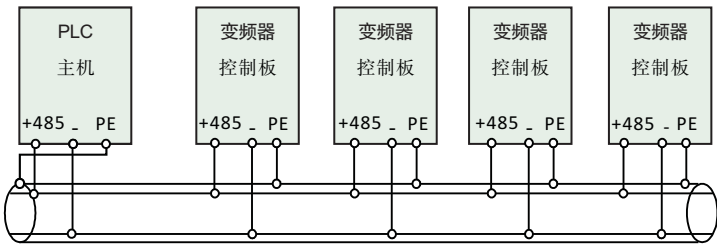
图3-12 PLC与变频器多机通信时的接线图（变频器、电机全部良好接地）
