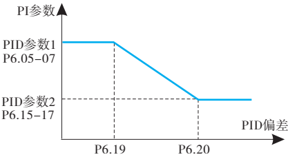
图6-27 PID参数切换
