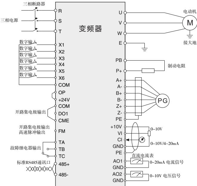
图3-4 0.75~3.7KW基本配线图
