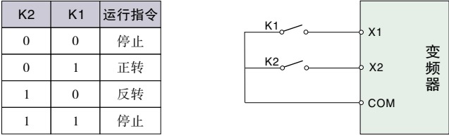
图6-19 两线式运转模式1
