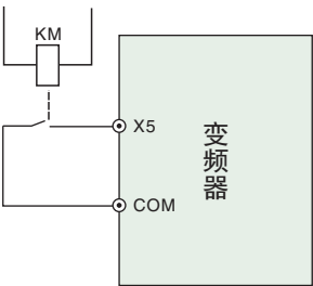
图6-17 外部设备故障输入示意图
