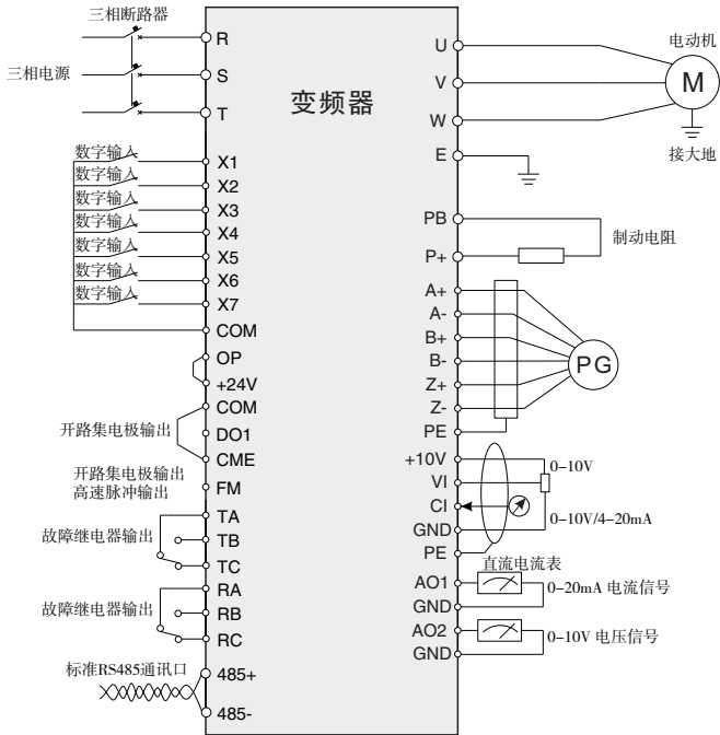
图3-5 5.5KW以上基本配线图
