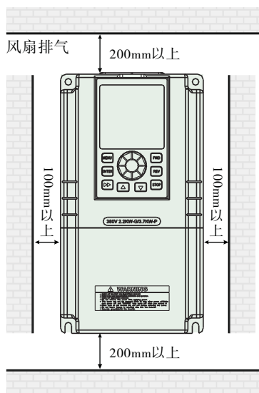
图 3-1 安装间隔距离示意图
