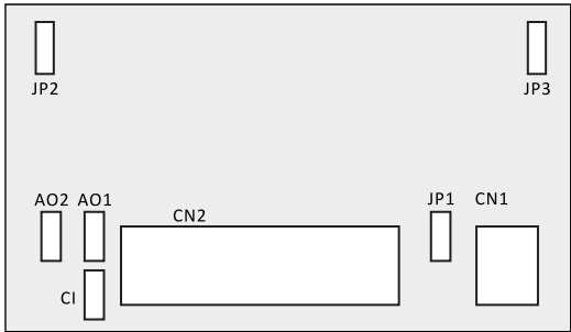
图3-6 控制板端子跳线位置示意图
